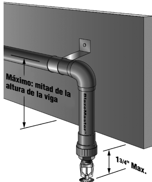
Líneas derivadas soportadas mediante colgador separador
