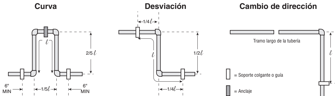
Figura 4: Configuración de curva y desviación de expansión
