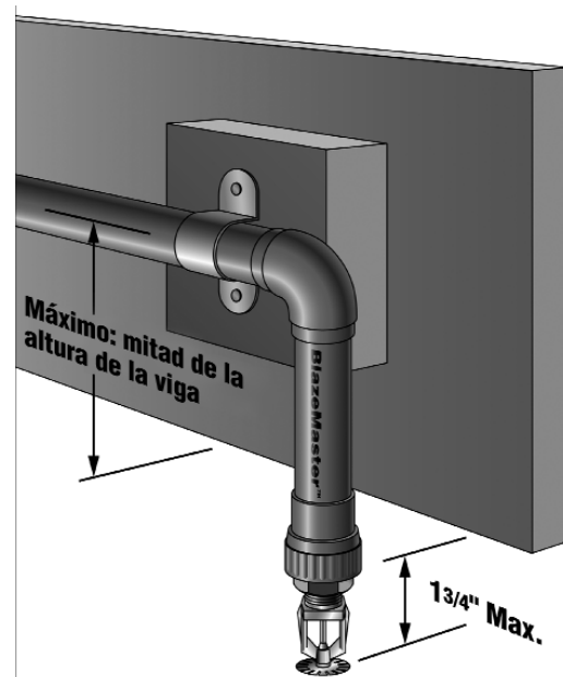
Líneas derivadas soportadas mediante bloques
